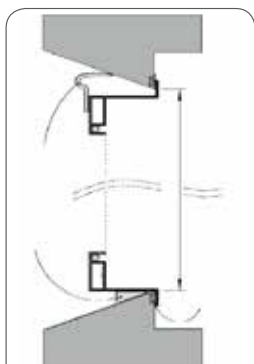
Type B Plastvindue -m/ lige int. sålbænk
