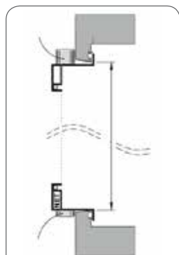
Type A Plastvindue -uden sålbænk
