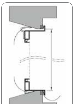
Type C Plastvindue -m/ knækket int. sålbænk
