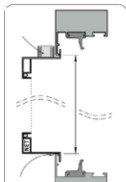
Type ALU Aluvindue -tynd karm kant
